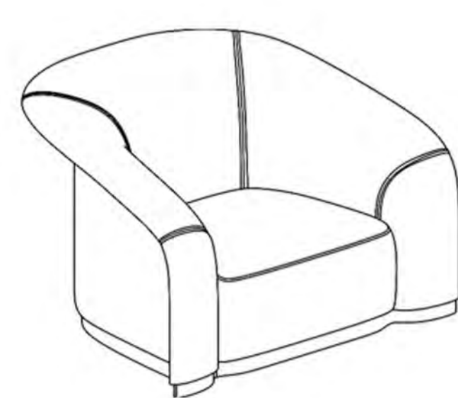
名称 NAME : 单人位 型号 MODEL : 21003-SF01 规格 SIZE : 1300(w)*1100(D)*840(H)mm
