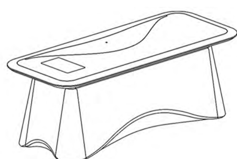
名称 NAME : 茶台 型号 MODEL : 21003-C22 规格 SIZE : 2200(w)*860(D)*776(H)mm
