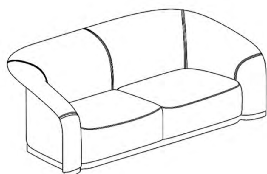
名称 NAME : 三人位沙发 型号 MODEL : 21003-SF03 规格 SIZE : 2400(w)*1100(D)*840(H)mm
